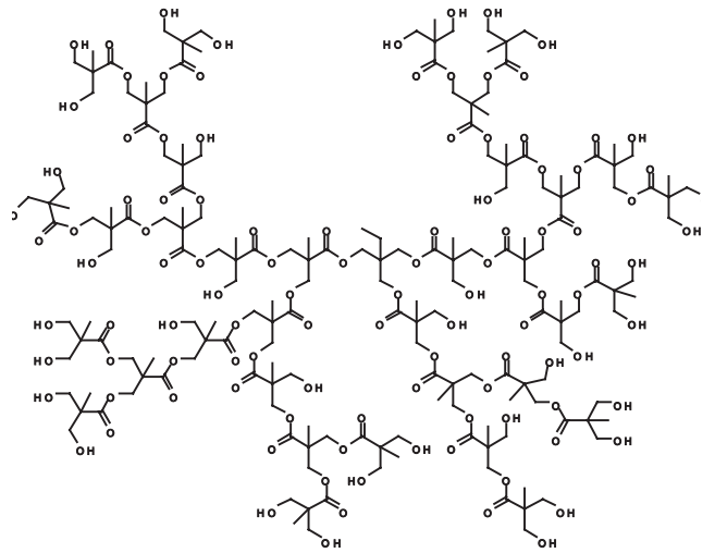
Dendritic polymer
